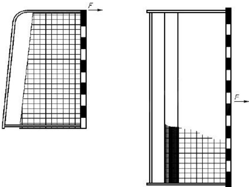
Рисунок 4 - Проверка стабильности ворот для мини-футбола
