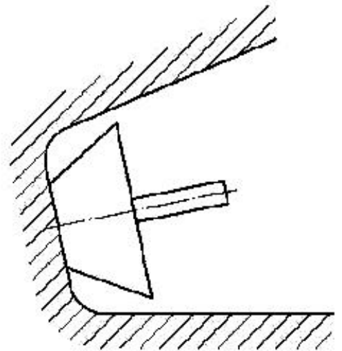
Рисунок 10 - Проверка соответствия оборудования требованиям к обеспечению предотвращения застреваний частей тела
