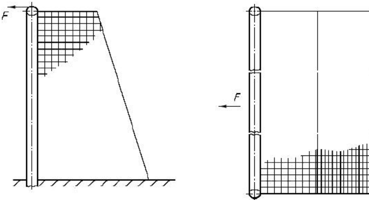
Рисунок 3 - Проверка стабильности ворот для футбола
