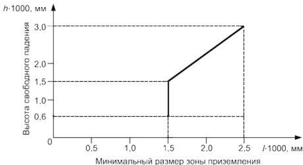
Рисунок 14 - Размеры зоны приземления
