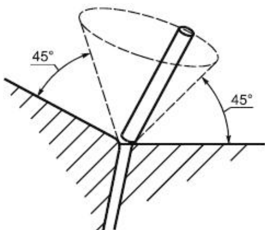
Рисунок Г.14 - Схема вращения стержня-пальца
