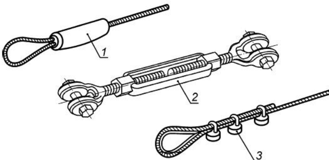
Рисунок 18 - Опрессованная петля, талреп, петля с коушем и зажимами
