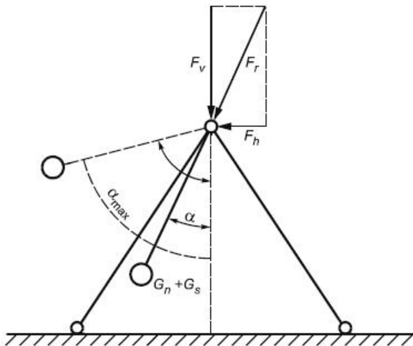
Рисунок А.2 - Силы, действующие на качели
