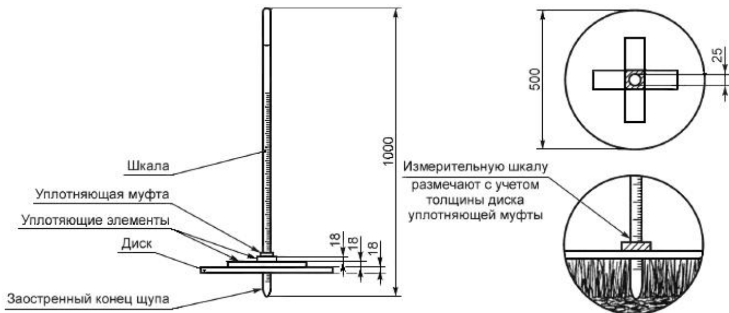
Рисунок 2 - Измерительный диск
