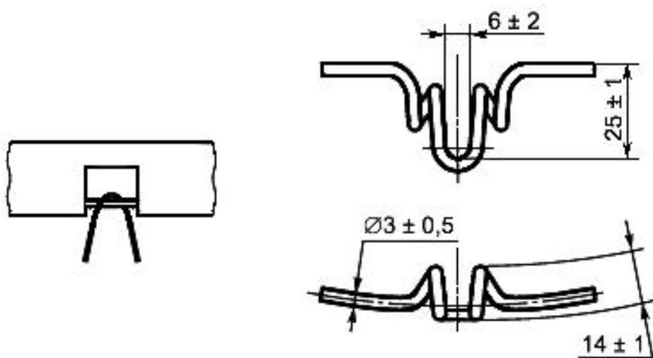
Рисунок 6 - Пример крючков для крепления сетки
