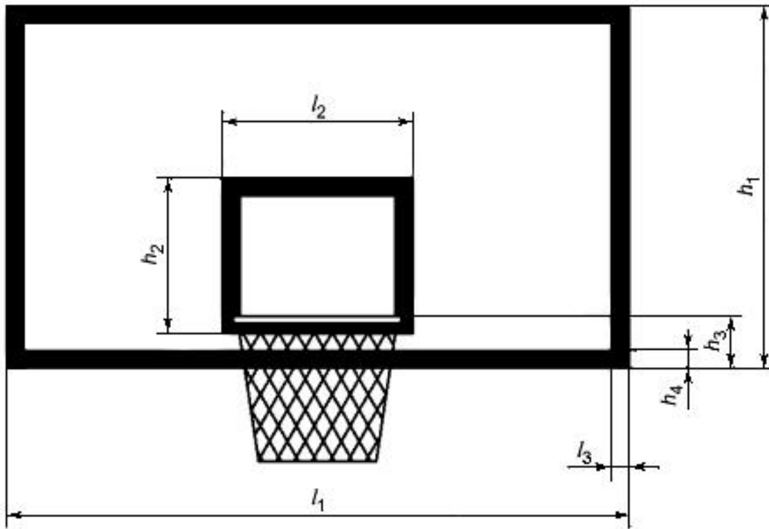
Рисунок 3 - Размеры и разметка баскетбольного щита
