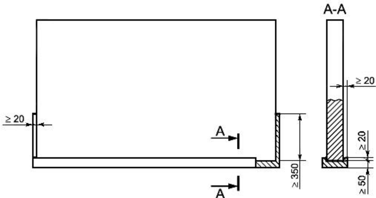
Рисунок 7 - Обивка баскетбольных щитов и стоек
